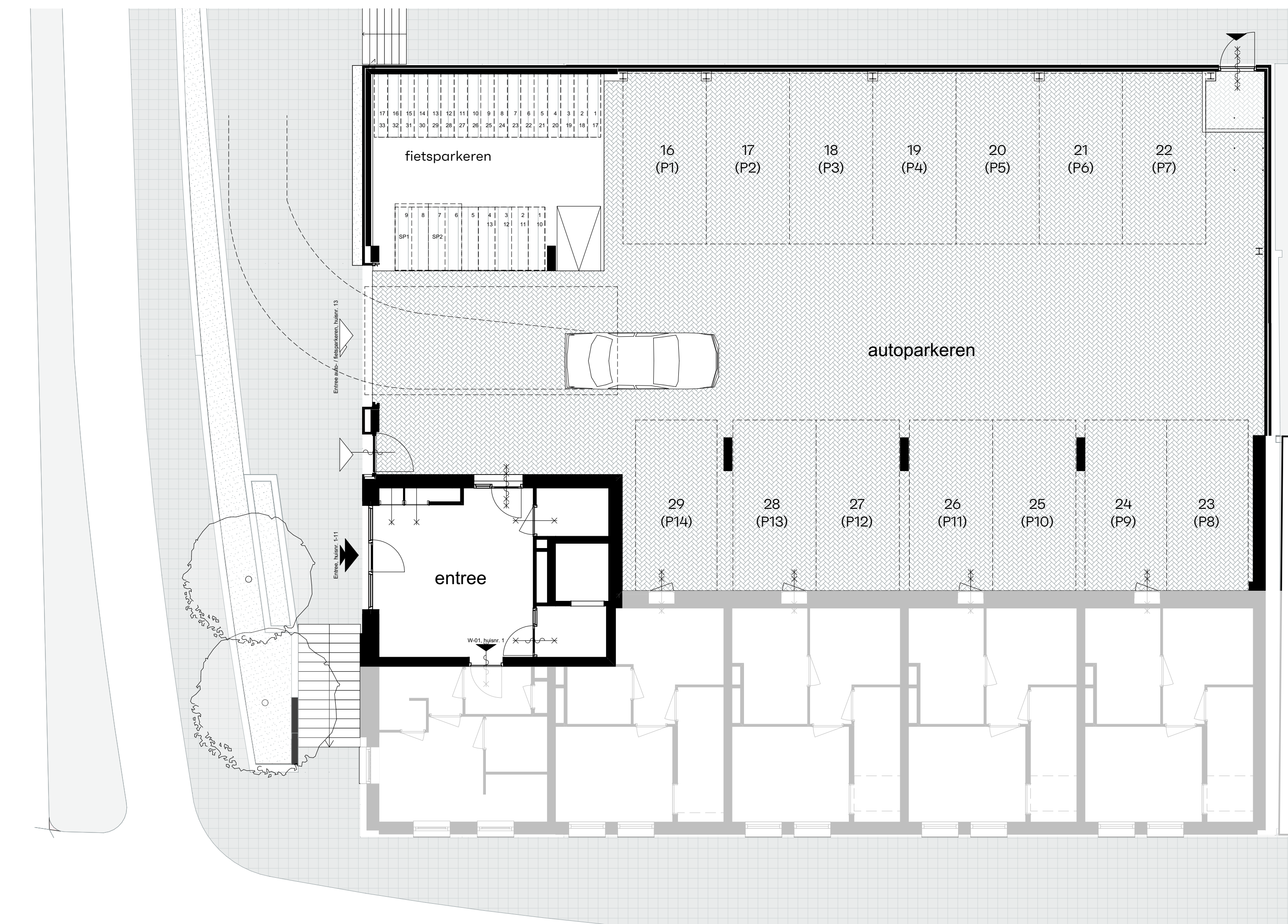
1:100 Souterrain overzicht
