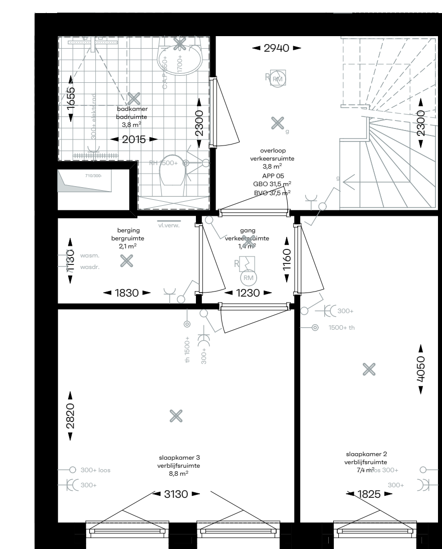
1:50 1e verdieping
