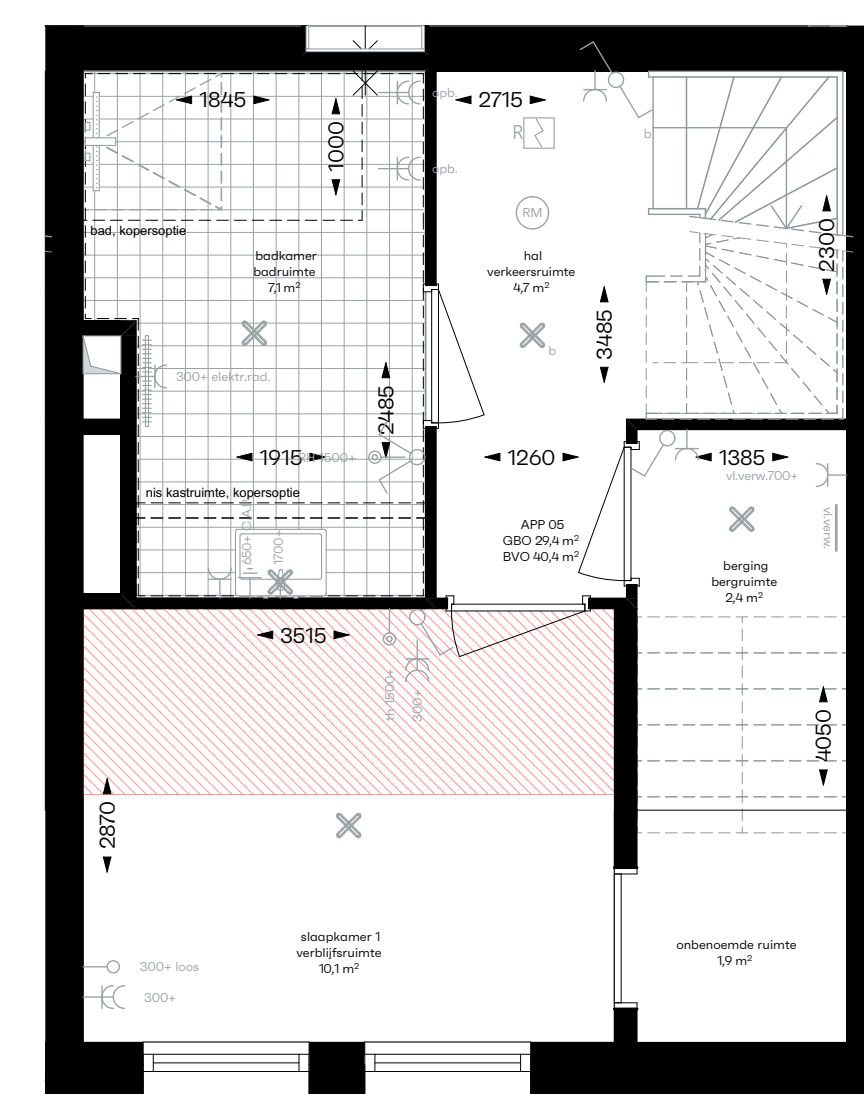
1:50 Souterrain
